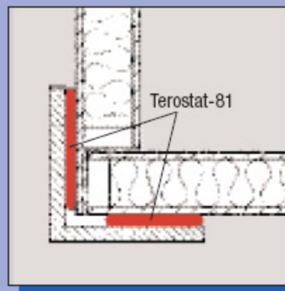
Uszczelnianie segmentów wzdłużnych
